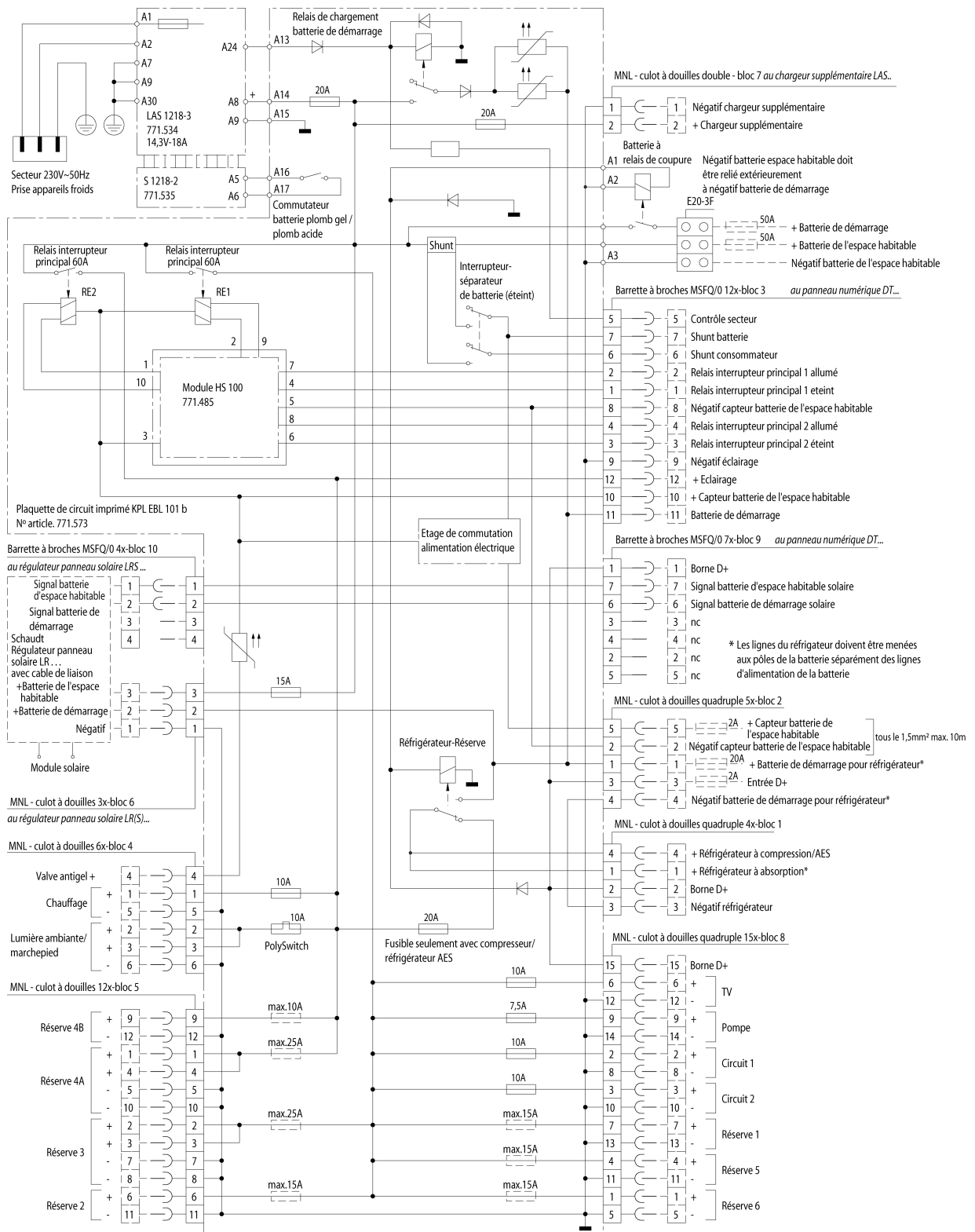
Fig. 2 Schéma fonctionnel bloc électrique EBL 101
