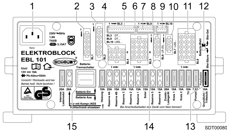
Fig. 1 Vue frontale du bloc électrique EBL 101
